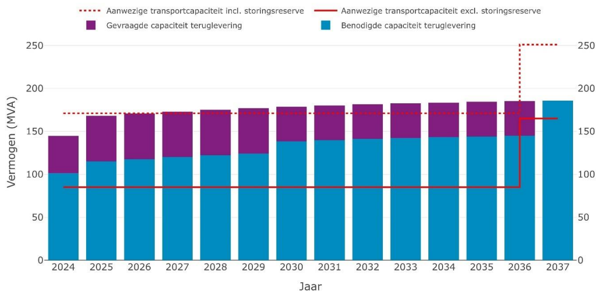
Figuur 2: Ontwikkeling van de aanwezig transportcapaciteit op congestiegebied Borculo tot en met het eerste kwartaal van 2036
