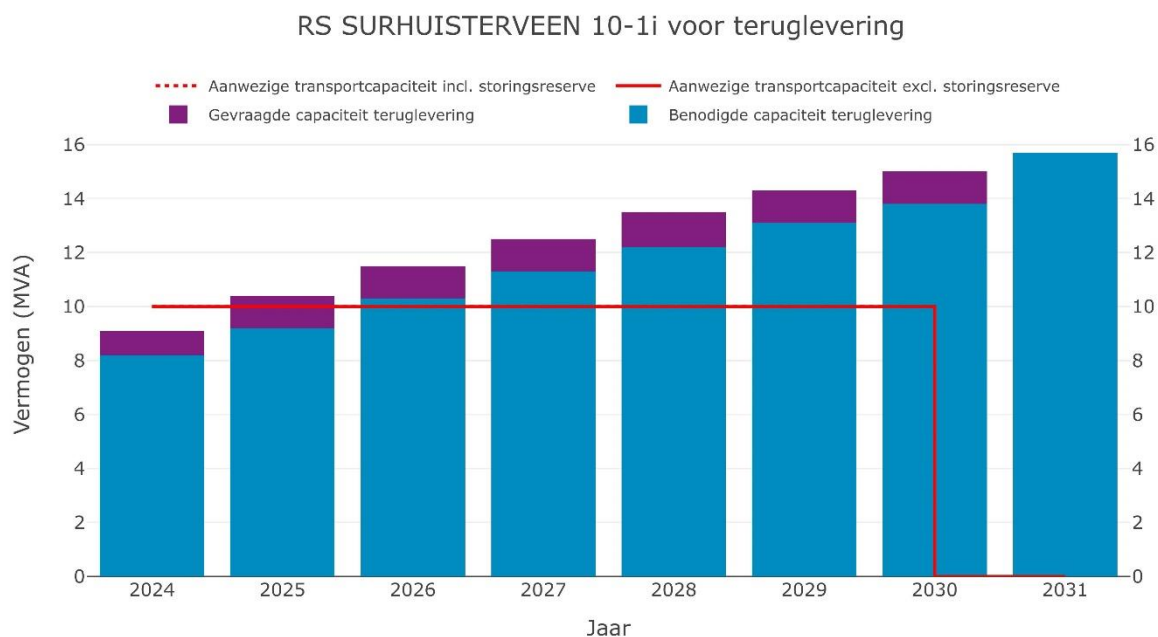
Figuur 2: Ontwikkeling van de aanwezig transportcapaciteit op congestiegebied Surhuisterveen tot en met het eerste kwartaal van 2030
