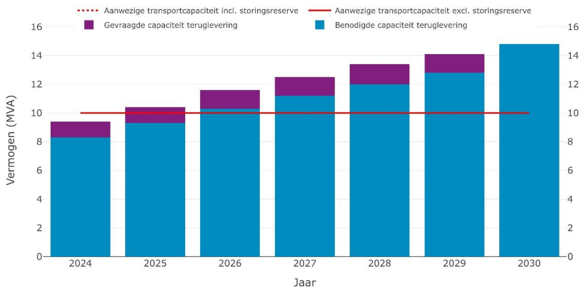
Figuur 3: Ontwikkeling van de aanwezig transportcapaciteit op congestiegebied Rijperkerk tot en met het tweede kwartaal van 2029
