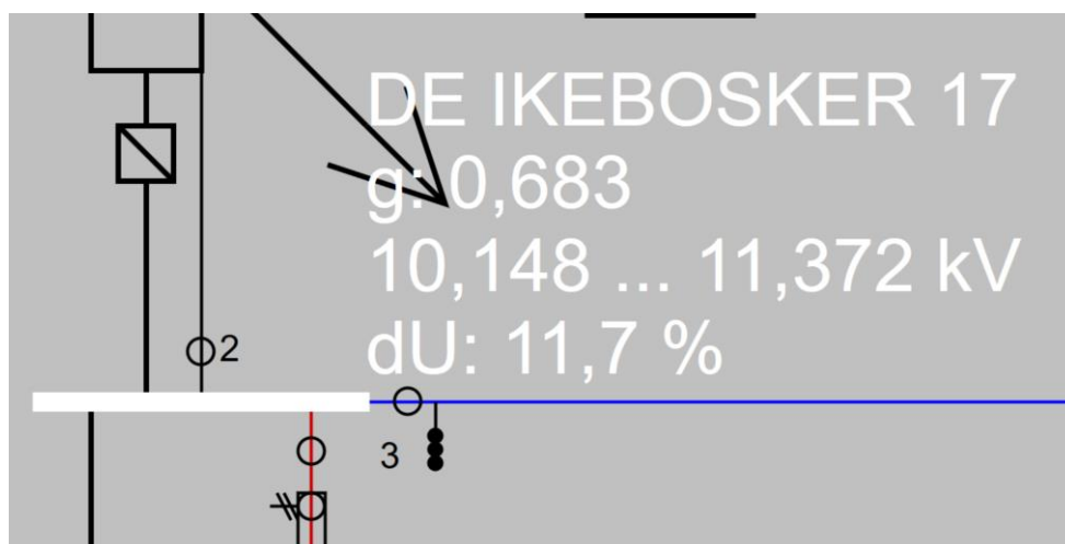
Figuur 3: Locatie met de slechtste spanning resultaten welke buiten de beleidsgrenzen vallen
