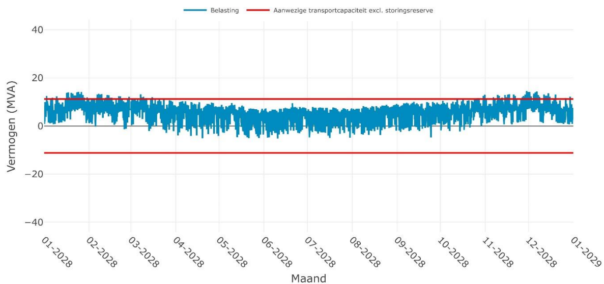
Verwachte belasting op SS MONNICKENDAM 10-1i voor het jaar 2028
