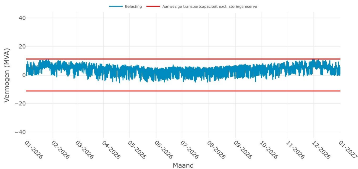
Verwachte belasting op SS MONNICKENDAM 10-1i voor het jaar 2026
