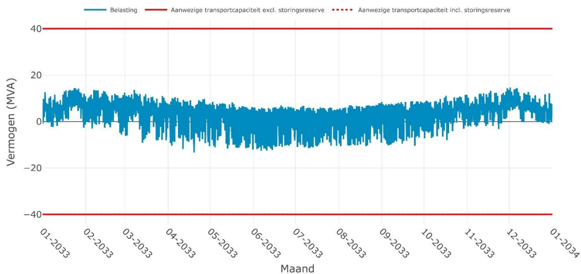
Verwachte belasting op SS MONNICKENDAM 10-1i voor het jaar 2033
