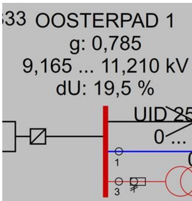
Figuur 5: Locatie met slechtste spanningsresultaten welke buiten de beleidsgrenzen vallen
