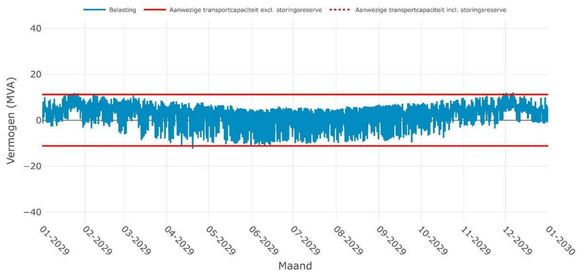
Verwachte belasting op SS MONNICKENDAM 10-1i voor het jaar 2029
