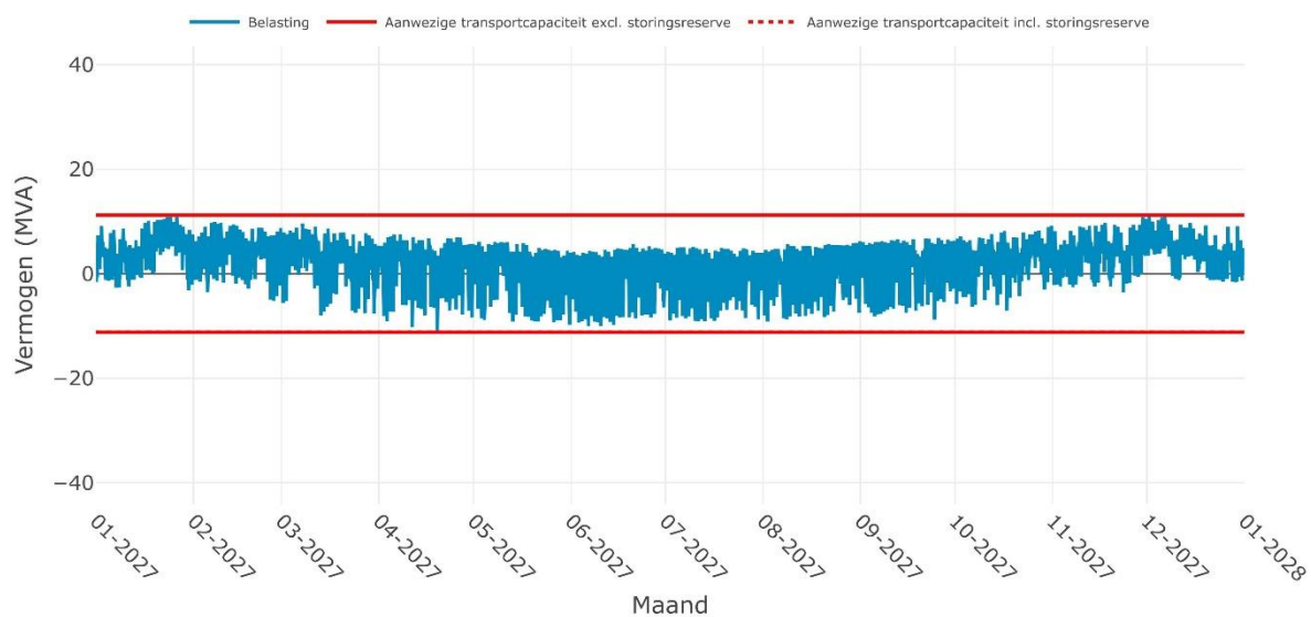
Verwachte belasting op SS MONNICKENDAM 10-1i voor het jaar 2027
