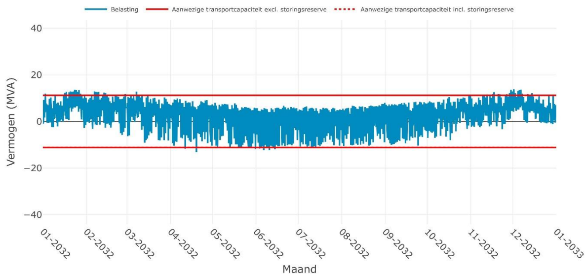
Verwachte belasting op SS MONNICKENDAM 10-1i voor het jaar 2032
