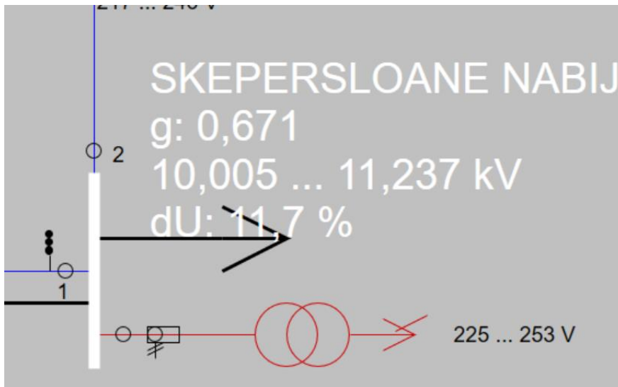
Figuur 4: Locatie met slechtste spanningsresultaten welke buiten de beleidsgrenzen vallen
