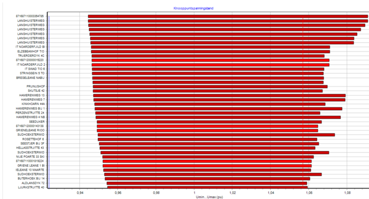
Figuur 2: Spanningscongestie
