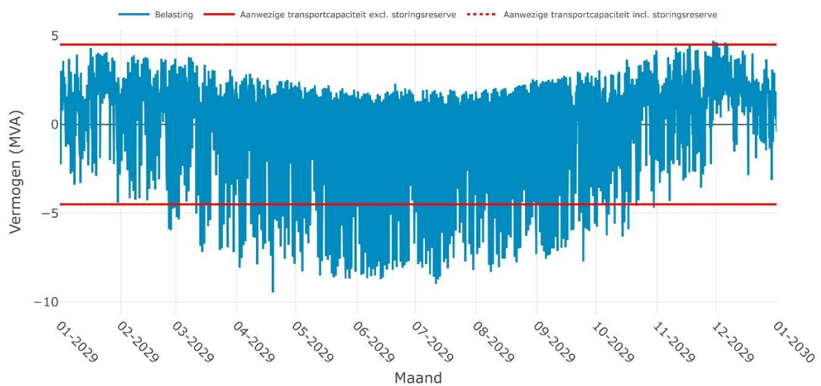
Verwachte belasting op SS WOMMELS 10-2i voor het jaar 2029
