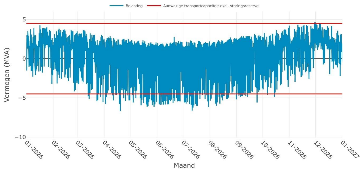
Verwachte belasting op SS WOMMELS 10-2i voor het jaar 2026
