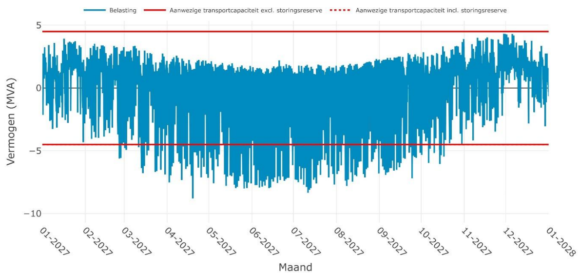
Verwachte belasting op SS WOMMELS 10-2i voor het jaar 2027
