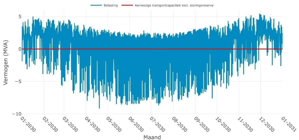
Verwachte belasting op SS WOMMELS 10-2i voor het jaar 2030
