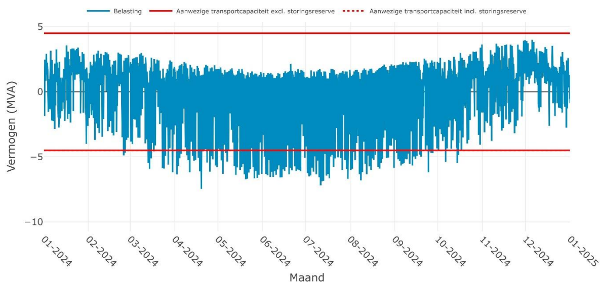
Verwachte belasting op SS WOMMELS 10-2i voor het jaar 2024
