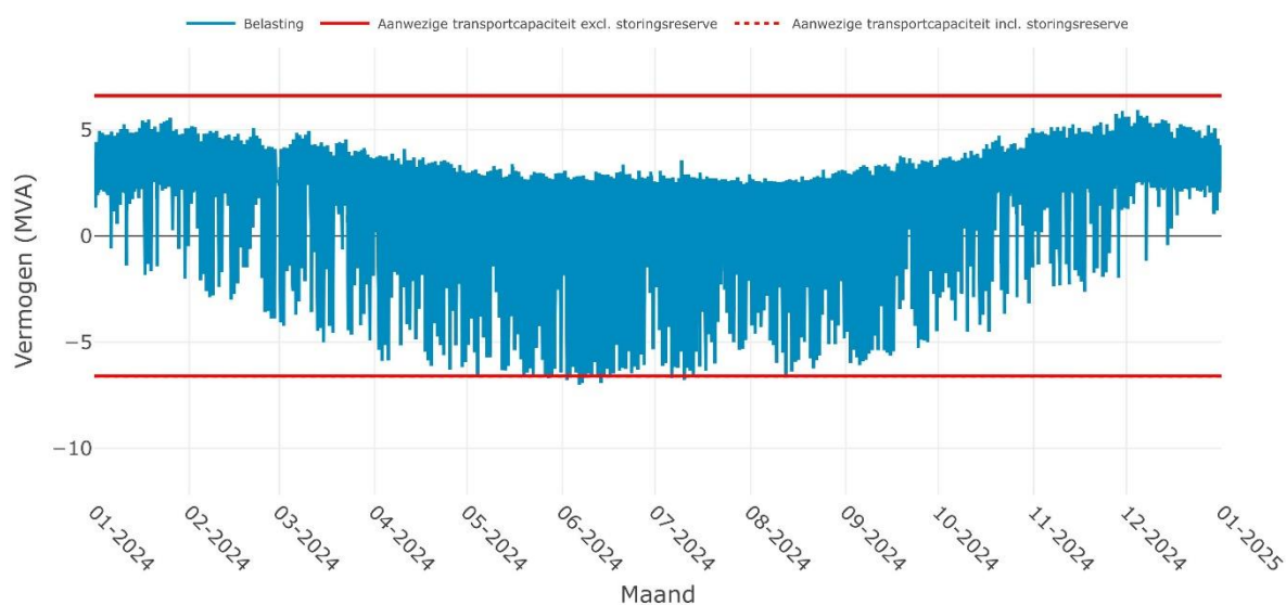
Verwachte belasting op SS HET HOP 10-1i + 10-2i voor het jaar 2024
