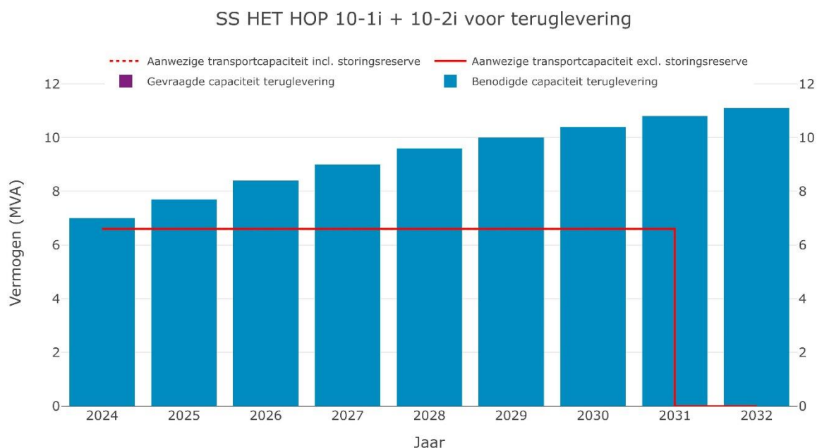
Figuur 2: Ontwikkeling van de aanwezig transportcapaciteit op Congestiegebied Het Hop tot en met het vierde kwartaal van 2030
