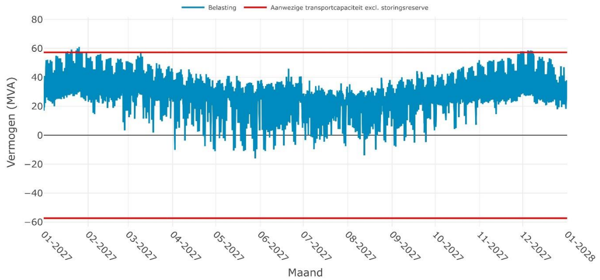
Verwachte belasting op OS LEEUWARDEN 10-4i voor het jaar 2027
