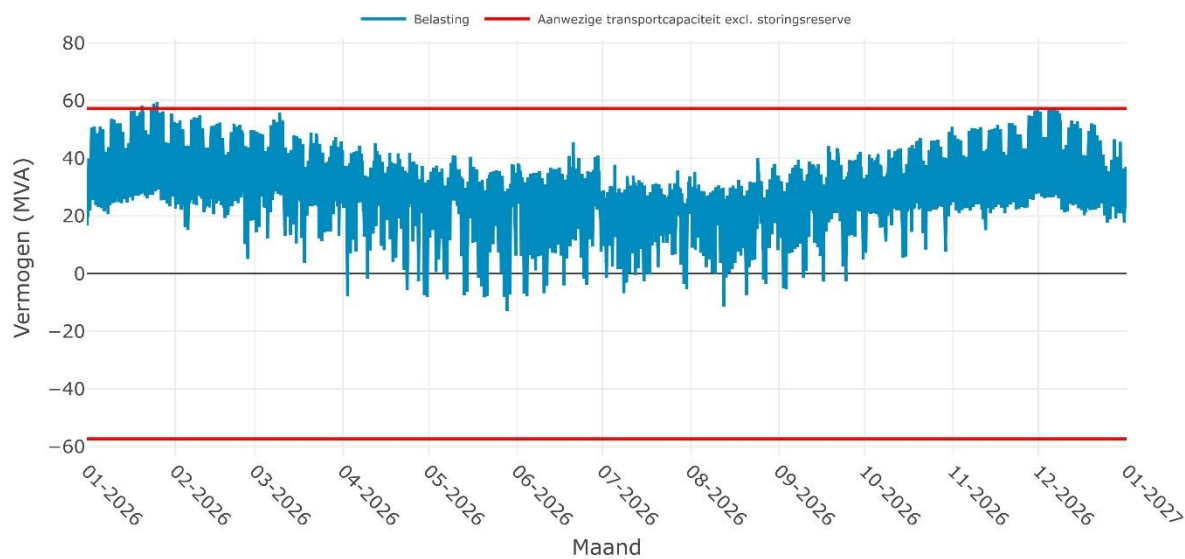
Verwachte belasting op OS LEEUWARDEN 10-4i voor het jaar 2026
