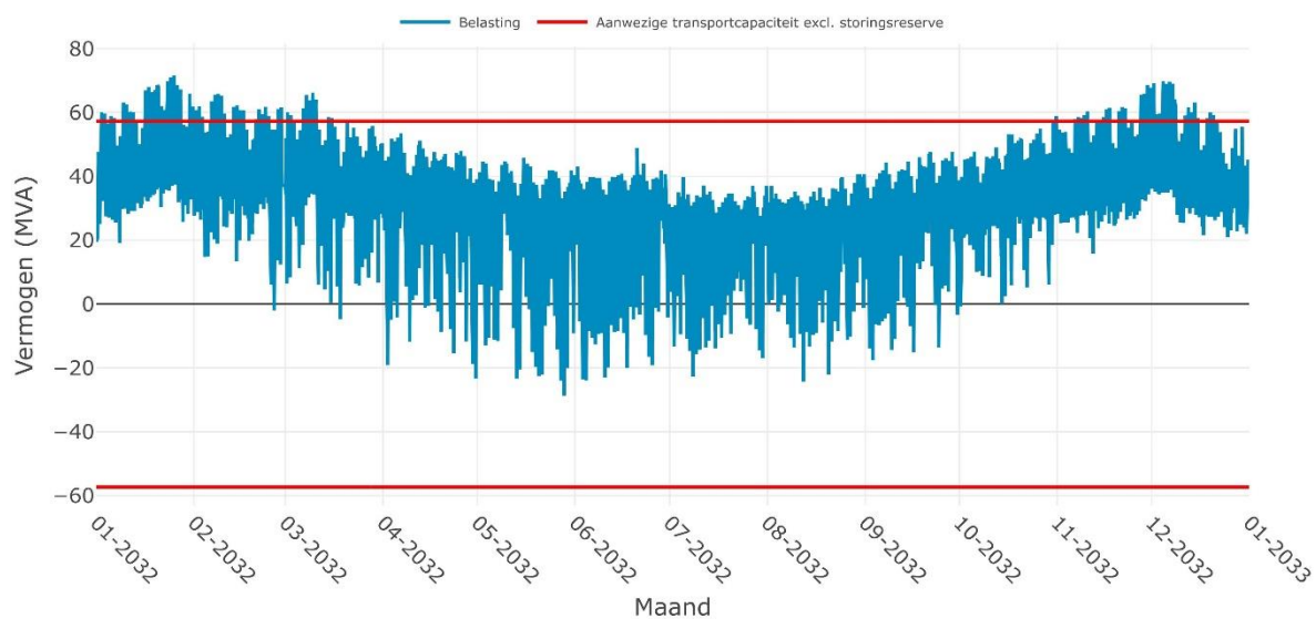
Verwachte belasting op OS LEEUWARDEN 10-4i voor het jaar 2032
