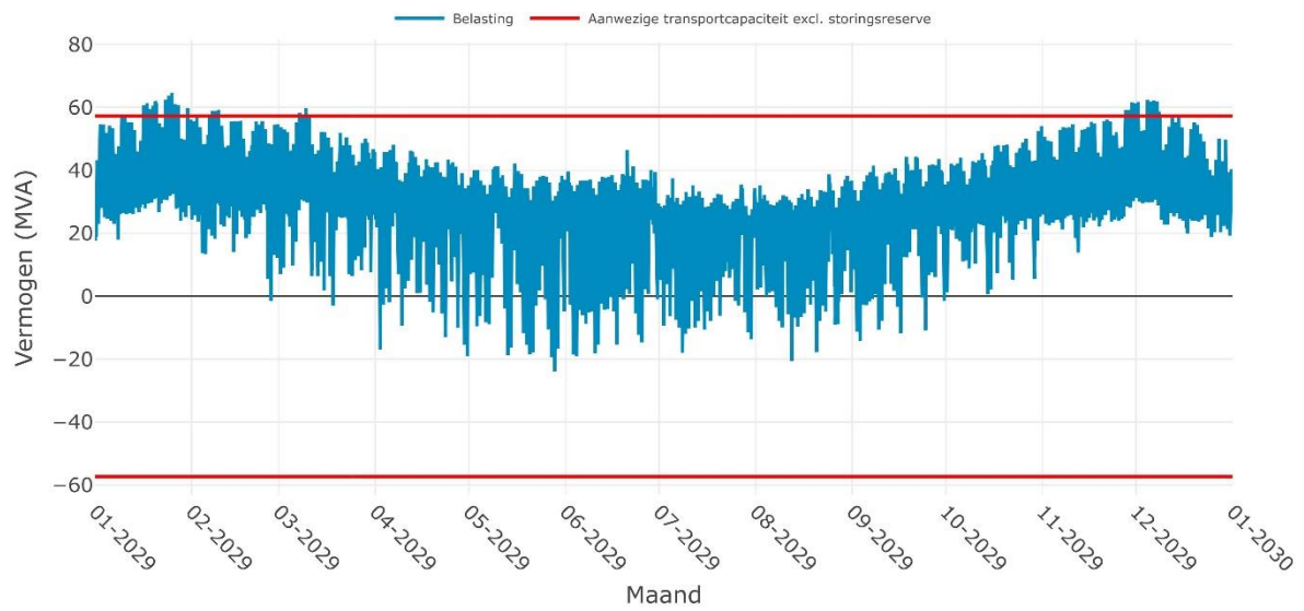
Verwachte belasting op OS LEEUWARDEN 10-4i voor het jaar 2029
