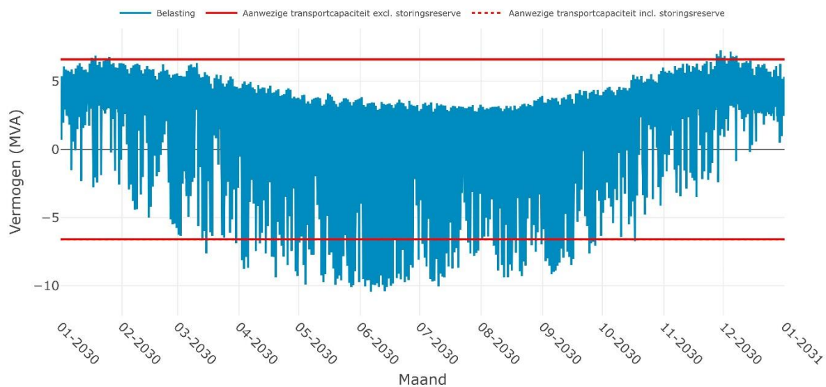
Verwachte belasting op SS HET HOP 10-1i + 10-2i voor het jaar 2030
