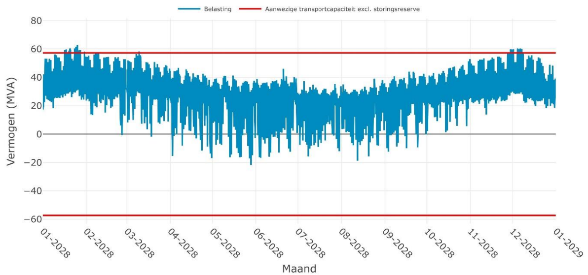
Verwachte belasting op OS LEEUWARDEN 10-4i voor het jaar 2028
