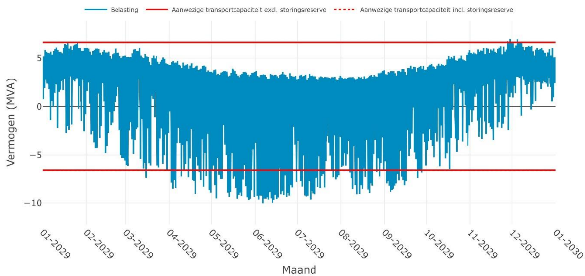
Verwachte belasting op SS HET HOP 10-1i + 10-2i voor het jaar 2029
