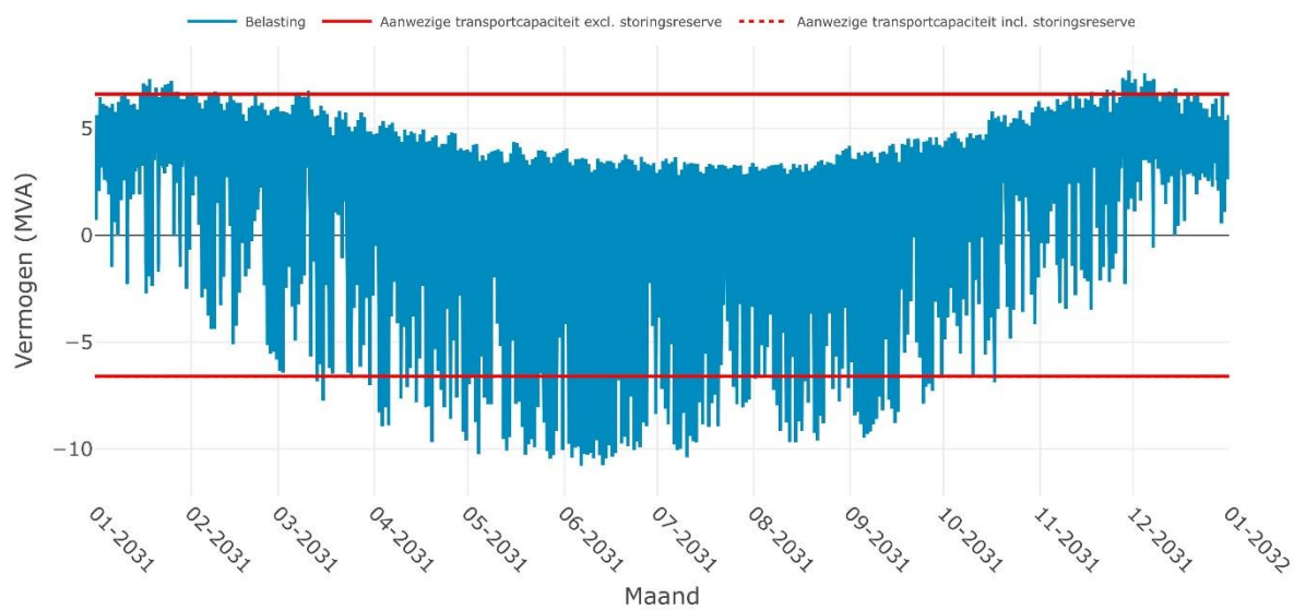
Verwachte belasting op SS HET HOP 10-1i + 10-2i voor het jaar 2031
