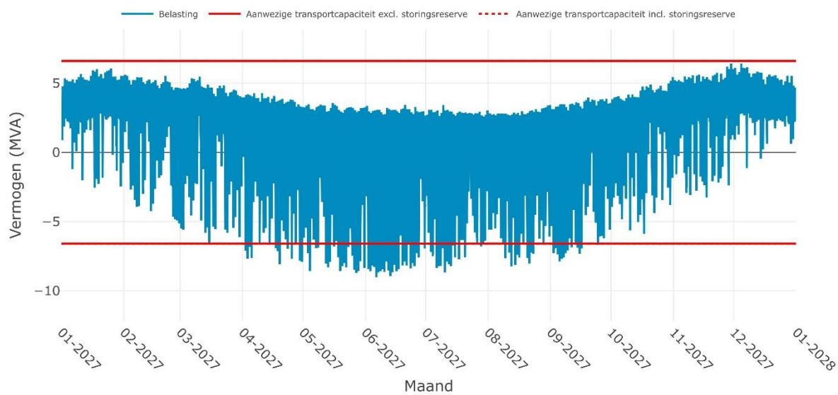
Verwachte belasting op SS HET HOP 10-1i + 10-2i voor het jaar 2027
