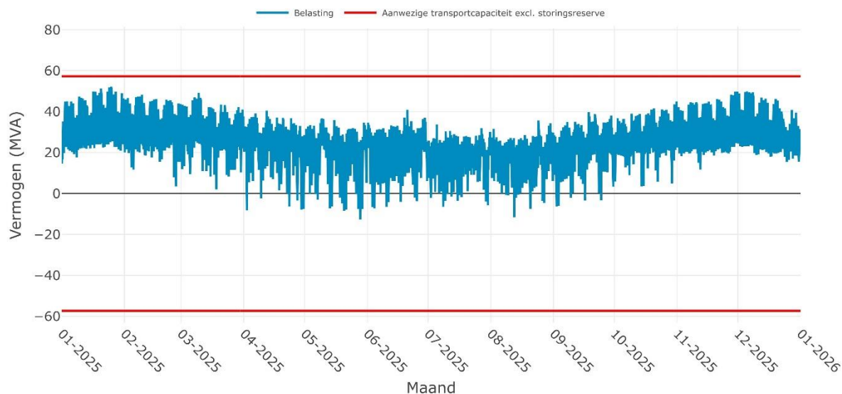
Verwachte belasting op OS LEEUWARDEN 10-4i voor het jaar 2025
