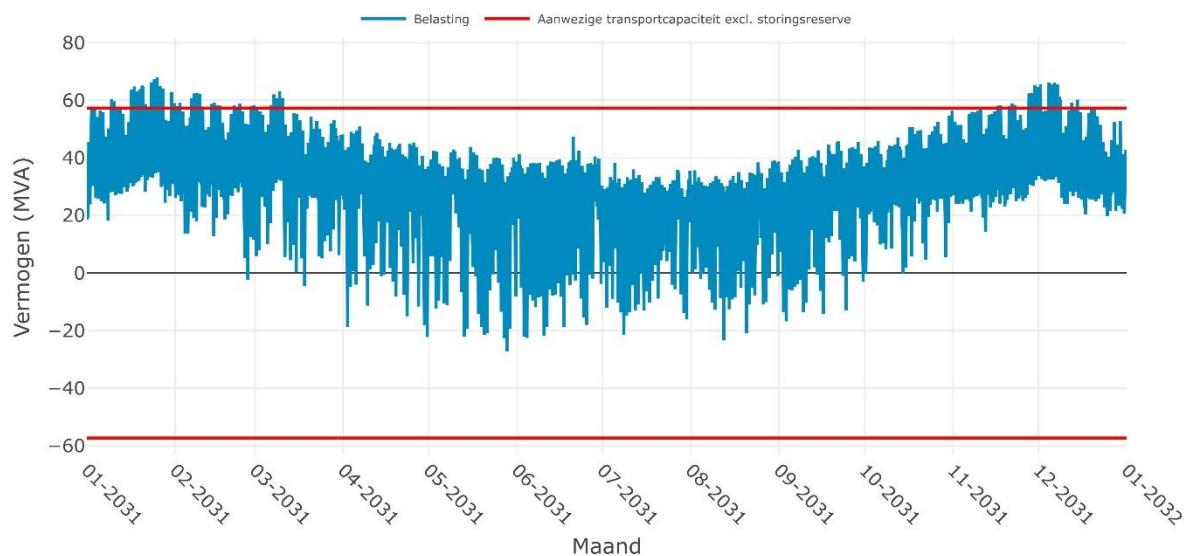
Verwachte belasting op OS LEEUWARDEN 10-4i voor het jaar 2031
