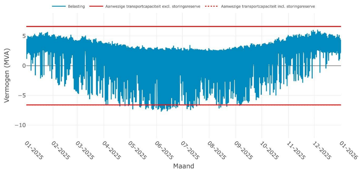
Verwachte belasting op SS HET HOP 10-1i + 10-2i voor het jaar 2025
