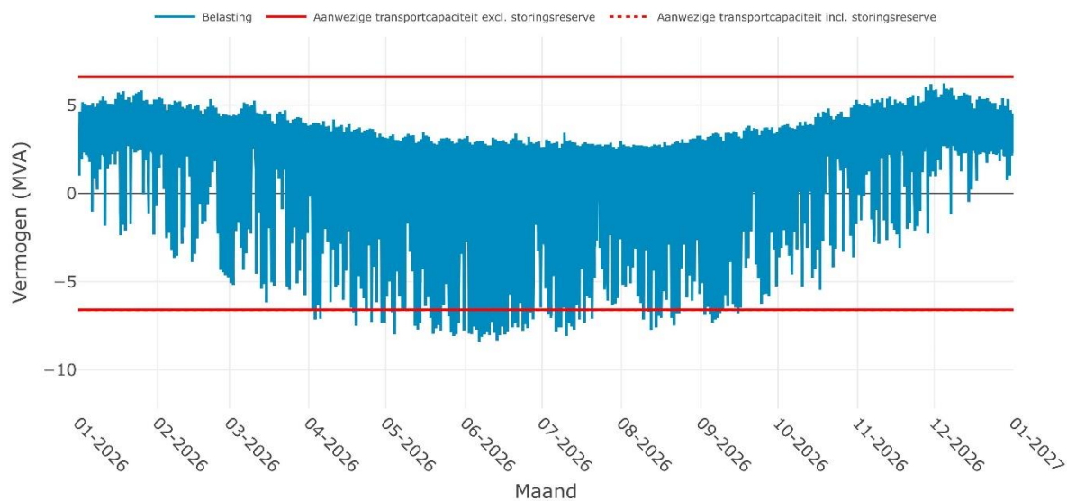
Verwachte belasting op SS HET HOP 10-1i + 10-2i voor het jaar 2026
