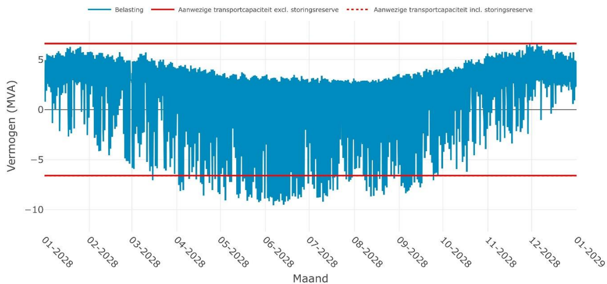
Verwachte belasting op SS HET HOP 10-1i + 10-2i voor het jaar 2028
