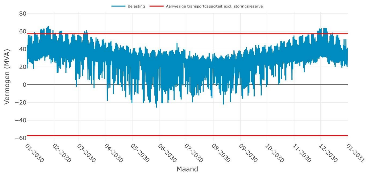
Verwachte belasting op OS LEEUWARDEN 10-4i voor het jaar 2030
