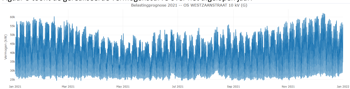
Figuur 3: Gerealiseerde vermogenscurve in het afgelopen jaar bij verdeelstation Westzaanstraat .
