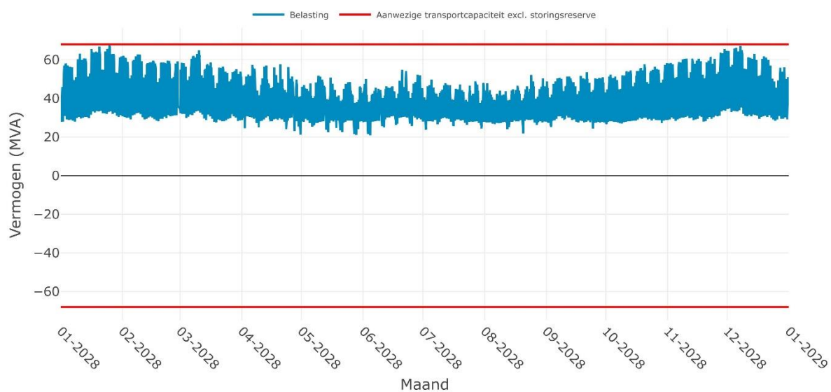
Verwachte belasting op OS WESTZAANSTRAAT 10-1i voor het jaar 2028
