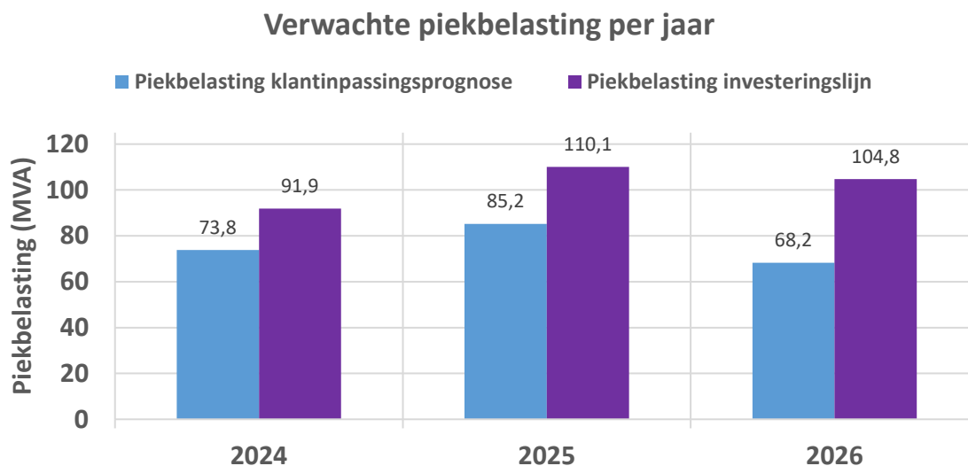
Figuur 3: Verwachte piekbelasting op verdeelstation Westhaven tot en met 2025.
