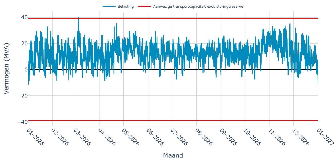
Verwachte belasting op OS WESTHAVEN 10-2i voor het jaar 2026
