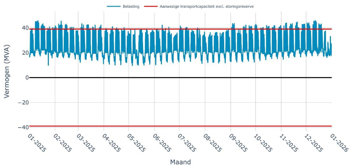
Verwachte belasting op OS WESTHAVEN 10-1i voor het jaar 2025
