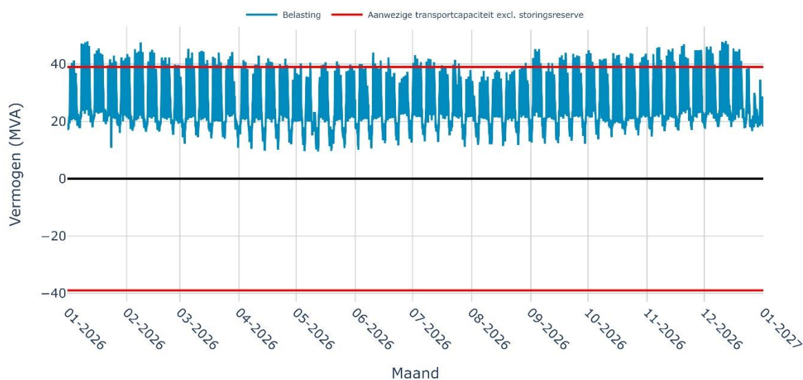
Verwachte belasting op OS WESTHAVEN 10-1i voor het jaar 2026
