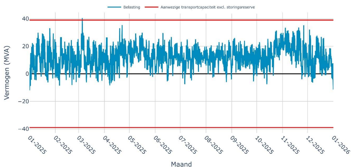
Verwachte belasting op OS WESTHAVEN 10-2i voor het jaar 2025
