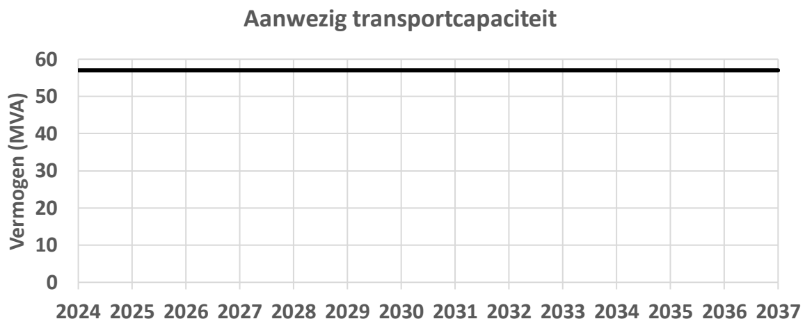
Figuur 2: Ontwikkeling van aanwezige transportcapaciteit op verdeelstation Sneek.
