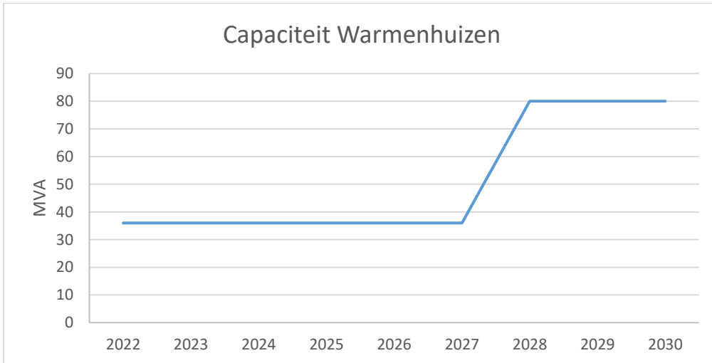
Figuur 7: Ontwikkeling van aanwezige transportcapaciteit in het congestiegebied.
